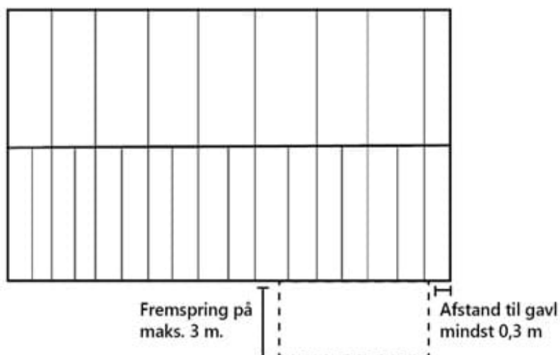
Principskitse for en mindre tilbygning ift. fremspring og afstand til gavl.
